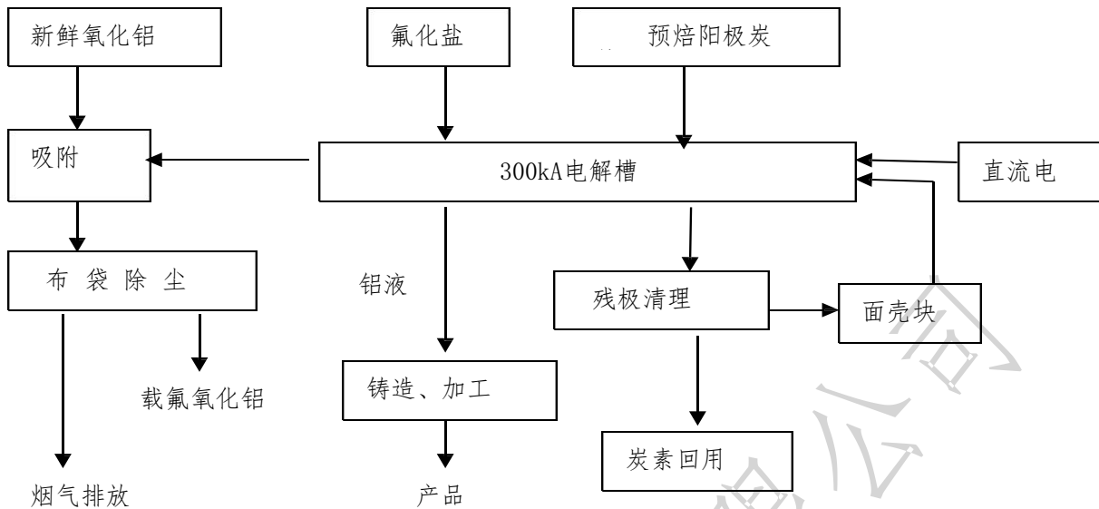
图 2 排放单位电解工艺流程图
