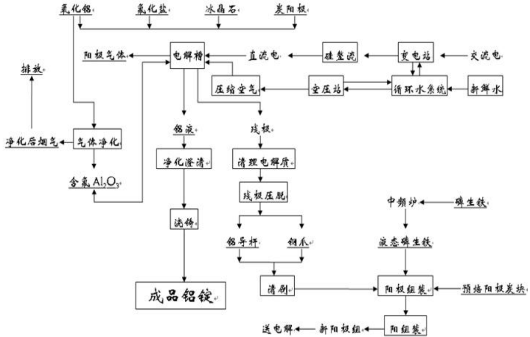
图 2 排放单位电解工艺流程图
