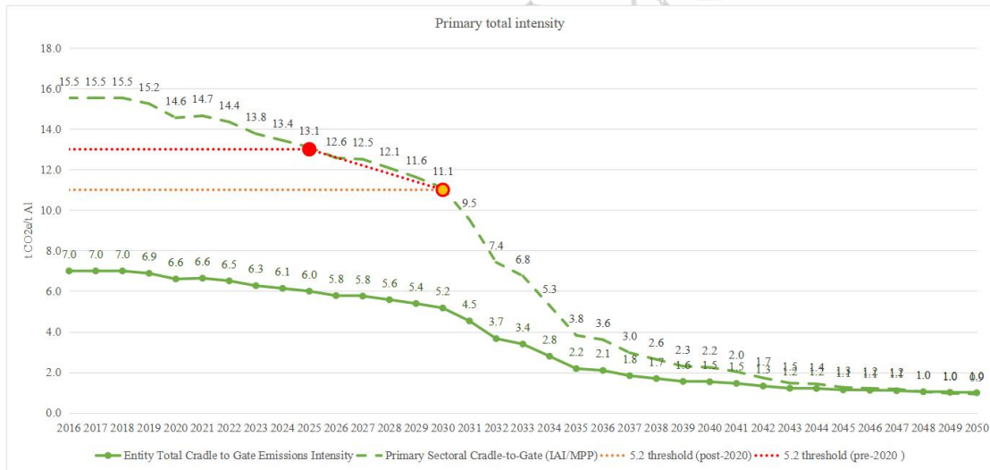
图 1 云铝涌鑫从矿山到金属铝铸锭的排放强度 1.5°C减排目标
