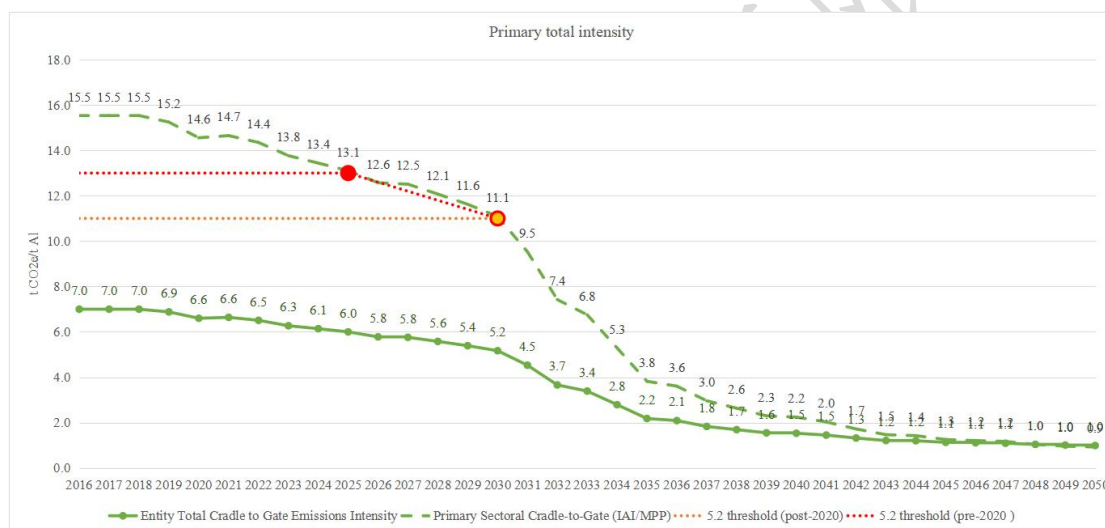
图 1 云铝润鑫从矿山到金属铝铸锭的排放强度 1.5°C减排目标
