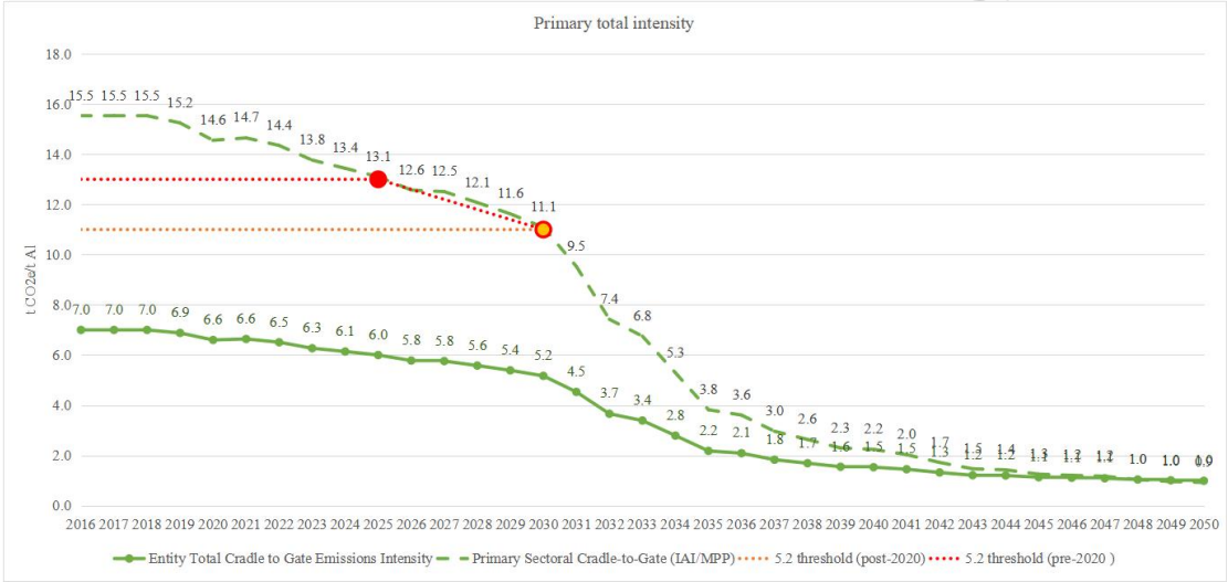
图 1 云铝润鑫从矿山到金属铝铸锭的排放强度 1.5℃减排目标
