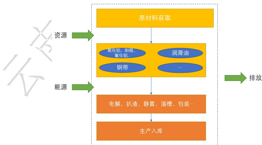
图 1 重熔用精铝锭生命周期系统边界
