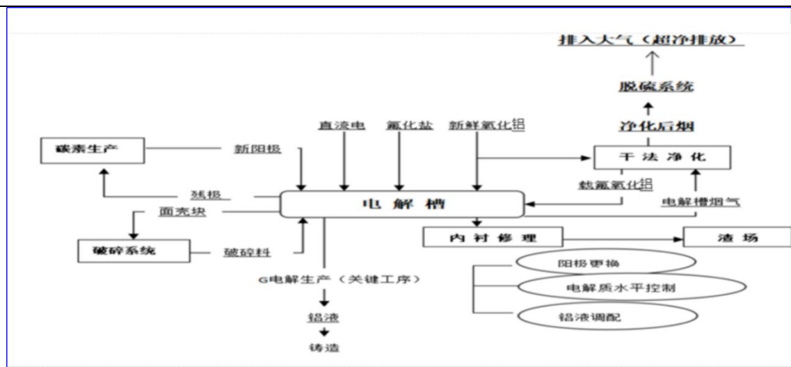
图2 电解铝液生产工艺流程图
