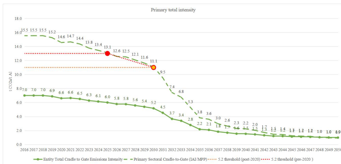
图 1 云铝涌鑫从矿山到金属铝铸锭的排放强度 1.5°C减排目标公司采用 ASI 温室气体减排路径工具 ASI-Entity-GHG-Pathways-Calculation-Tool (2025 年)，制定 1.5 摄氏度以下温升目标减排路径，确保温室气体减排途径符合全球温升控制在 1.5 摄氏度的情景要求。模型设定 2023 年为基准年，基础数据来源于《云南云铝涌鑫铝业有限公司 2023 年温室气体排放清单报告书》，范围 1+2 强度 0.02087 t CO 2 e/t Al，范围 3 (类别 1) 采购铝 (含废铝) 平均强度 6.2628 t CO 2 e/t Al，在模型中设置上述数据，得出 1.5 摄氏度以下温升目标减排路径如下图所示。
